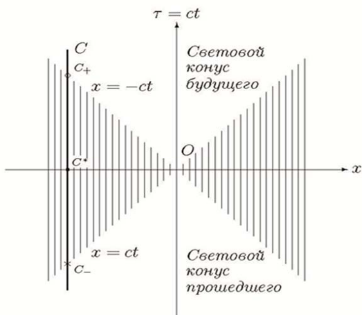
Рис. 1. Сечение светового конуса плоскостью (x, ct)
